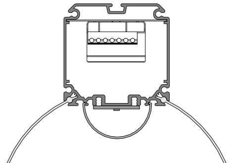
OPAL REFLECTOR LINEAR
